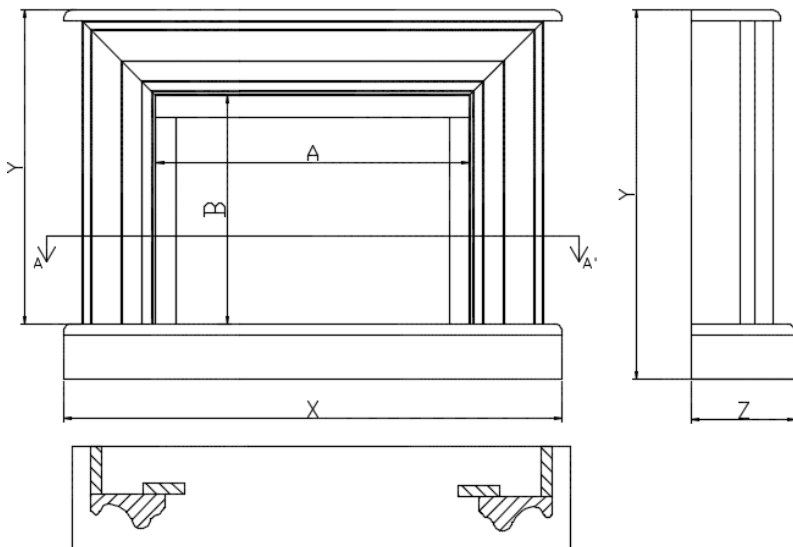
SECCIÓN A-A'
